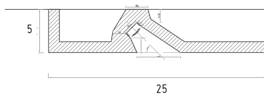
Profil lumineux D121 en 2 ml
