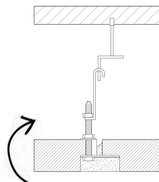
Vue en coupe du système de plafond (système breveté).
